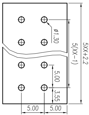
P.C.B. LAYOUT
