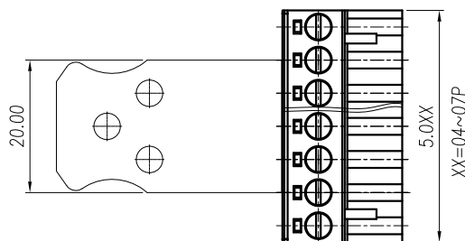
04~07P尺寸图
