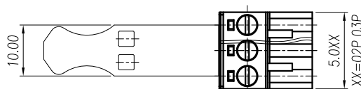
02~03P尺寸图
