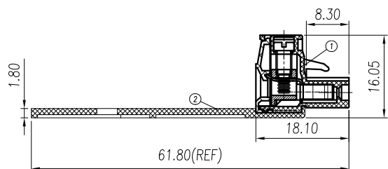
08~24P尺寸图
