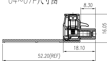
04~07P尺寸图
