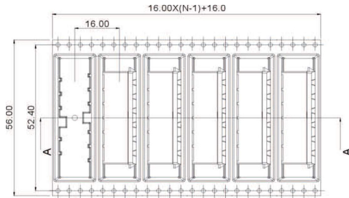
WJ2EDGV-THT-5.08
